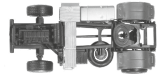
083676 Fahrgestell Zugmaschine 2achs MAN TGX/TGS Euro6c (2 Stück) / chassis rigid tractor 2axles (2 pieces)
