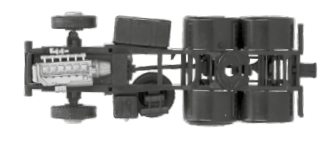
085793 H0 1:87 Fahrgestell Zugmaschine 3achs 8,95 € MAN/Roman Diesel, 2 Stück / chassis rigid tractor 3axle, 2 pieces
