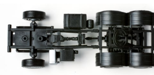
083485 H0 1:87 Fahrgestell Zugmaschine 3achs 9,95 € MAN TGX 6x6 Allrad (2 Stück) / chassis for tractor MAN 3-axle all-wheel (2 pieces)
