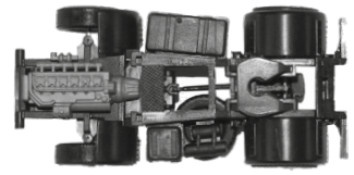
084925 H0 1:87 Fahrgestell Zugmaschine MAN 8,95 € F8, 2-achs, 2 Stück / Chassis rigid tractor, 2-axle, 2 pieces
