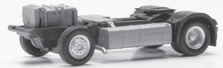
082716 Teileservice Fahrgestell Zugmaschine DAF XF 105 (2 Stück) H0 1:87 8,95 €
